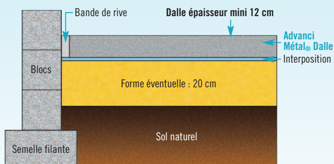
Coupe d'un dallage désolidarisé avec Advanci Métal® Dalle
