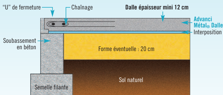
Dallage solidarisé de Maison Individuelle en Béton Renforcé de Fibres sous Avis Technique CSTB : Advanci Métal® Dalle
